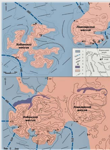
Распространение покровного льда в районе Хибинских и Ловозерских гор в периоды среднего (11.8 тыс. л. н.) (А) и позднего (10.3 тыс. л. н.) (Б) дриаса последнего оледенения. Из: Евзеров, 2015:127, рис. 152
